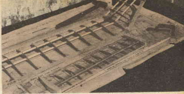
L'ala ed il piano di coda da rifinire, con le estremità ricavate da un blocchetto di balsa
