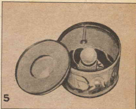
5 Veduta dell'interno della lampada da tavolo. Nel foro circolare al centro del coperchio va applicato il globetto di vetro il cui liquido provvede alla distribuzione della luce in modo indiretto
