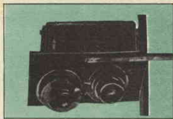
La macchina fotografica, trasformata per diminuirne il peso, e montata orizzontalmente. Osservare, a fianco dell'obiettivo, il « timer » ossia la sveglietta che al trascorrere del tempo per il quale era stata regolata fa scattare l'otturatore della macchina riprendendo la fotografia. L'obiettivo va regolato sull'infinito
