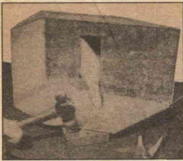
Foto a sinistra — Applicazione lungo i bordi del lamierino, di un filo di ferro o di ottone allo scopo di aumentare la resistenza della maschera alla deformazione. Il filo va saldato a stagno e poi, eventualmente su di esso va ribattuto il bordino del metallo, in modo da ovviare il pericolo che il margine tagliante di questo possa determinare ferite a chi inavvertitamente abbia la ventura di passarvi sopra la mano
