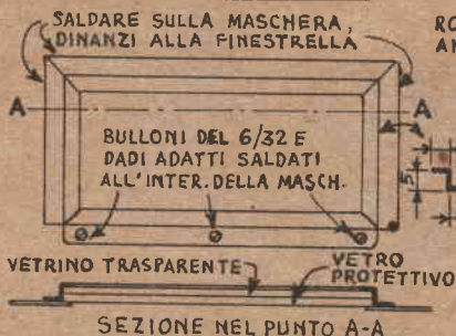
SEZIONE NEL PUNTO A-A
