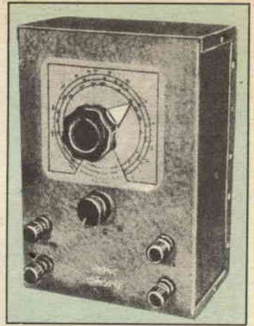
Veduta frontale dello strumento. In alto, il quadrante graduato, sotto ad esso il commutatore che inserisce la resistenza, il condensatore o l'induttanza campo, e a seconda del tipo di componente che interessa misurare. La coppia di morsetti a sinistra è quella ai quali va collegato il componente che interessa misurare mentre alla coppia di destra vanno collegate le cuffie di ascolto per il rilevamento dell'azzeramento.
