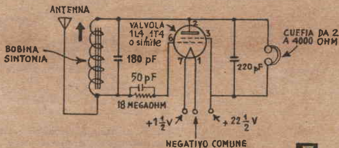
SCHEMA ELETTRICO
