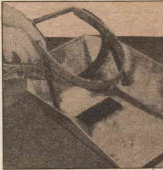
Foto a sinistra. — Costruzione della montatura che serve ad assicurare alla testa del saldatore, la maschera vera e propria; alcune delle strisce sono di fibra, altre sono invece di cuoio
